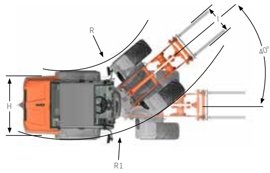
Mit Palettengabel
