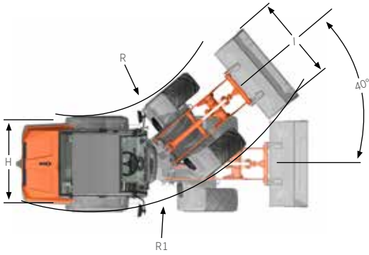
Mit Standardschaufel
